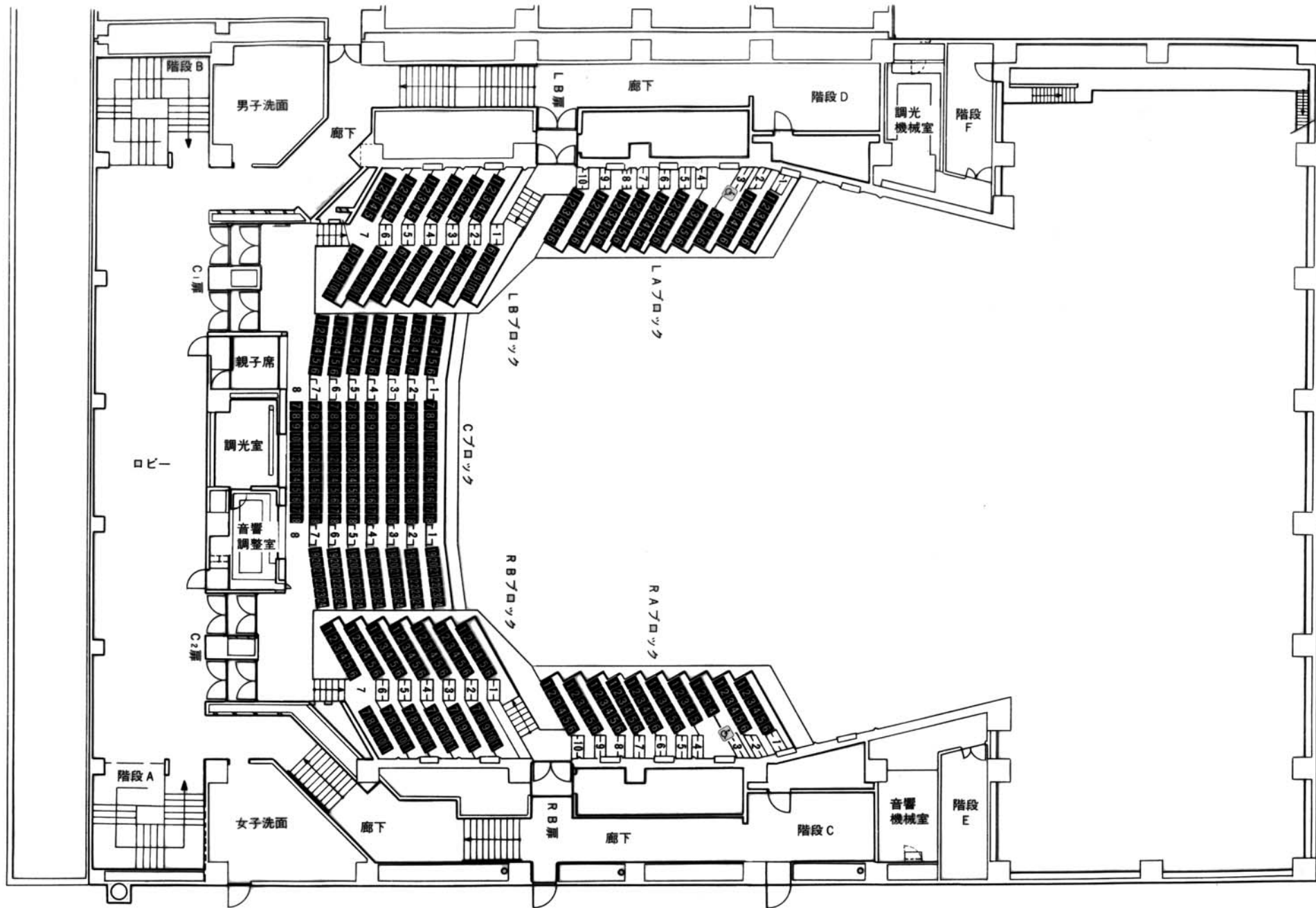
和光市民文化センター大ホール2F平面図
